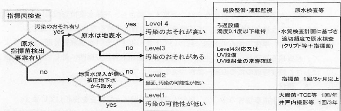
8 ■図表5-3 クリプトスポリジウム等対策のスキーム
