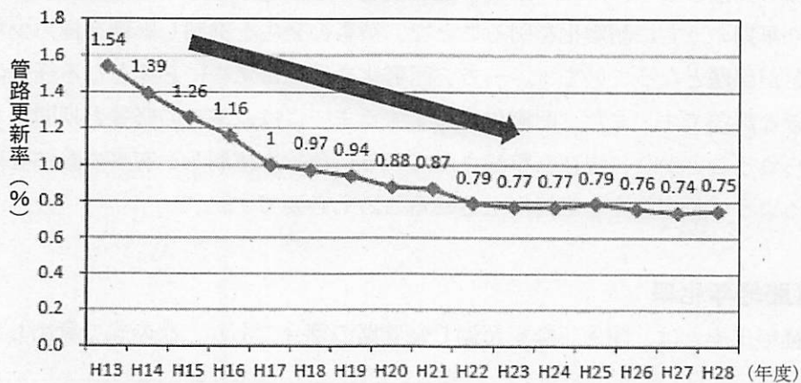
11 12 13 14 15 16 ■図表5-15 全国の管路更新率の推移
