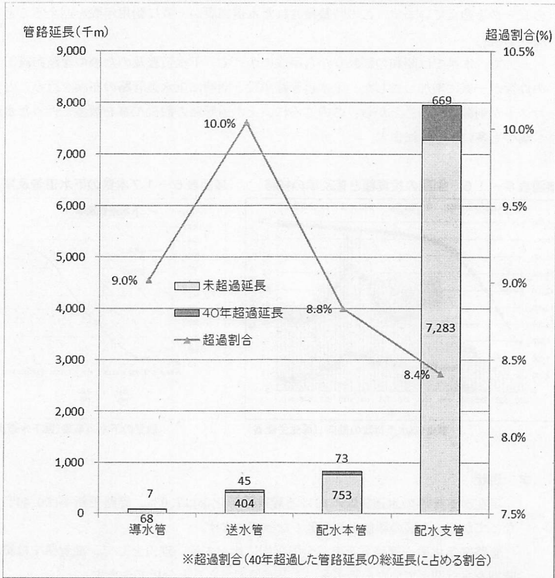
1 ■図表5-19 滋賀県の経年管路の延長と割合（上水道の基幹管路のみ）
