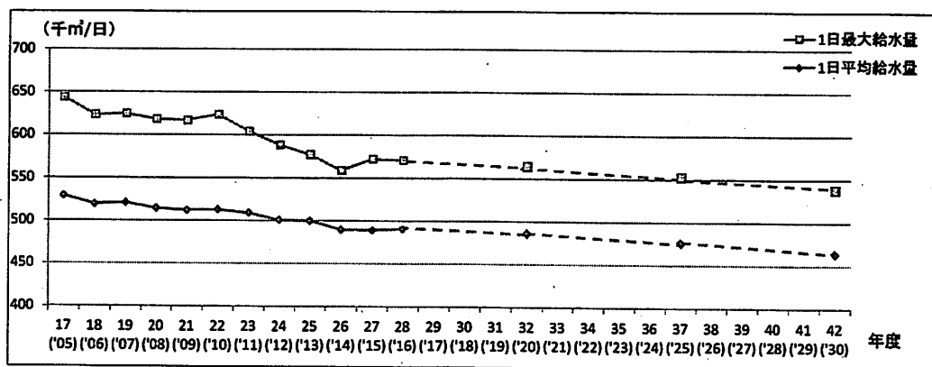
14 ■図表4-8 一日最大給水量および一日平均給水量の将来予測
