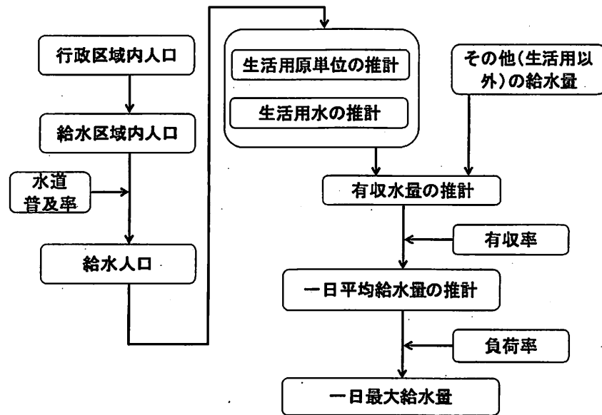
5 ■図表4-1 水需要予測フロー
