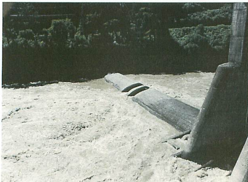
安曇川合同井堰 【エプロンの洗掘】
