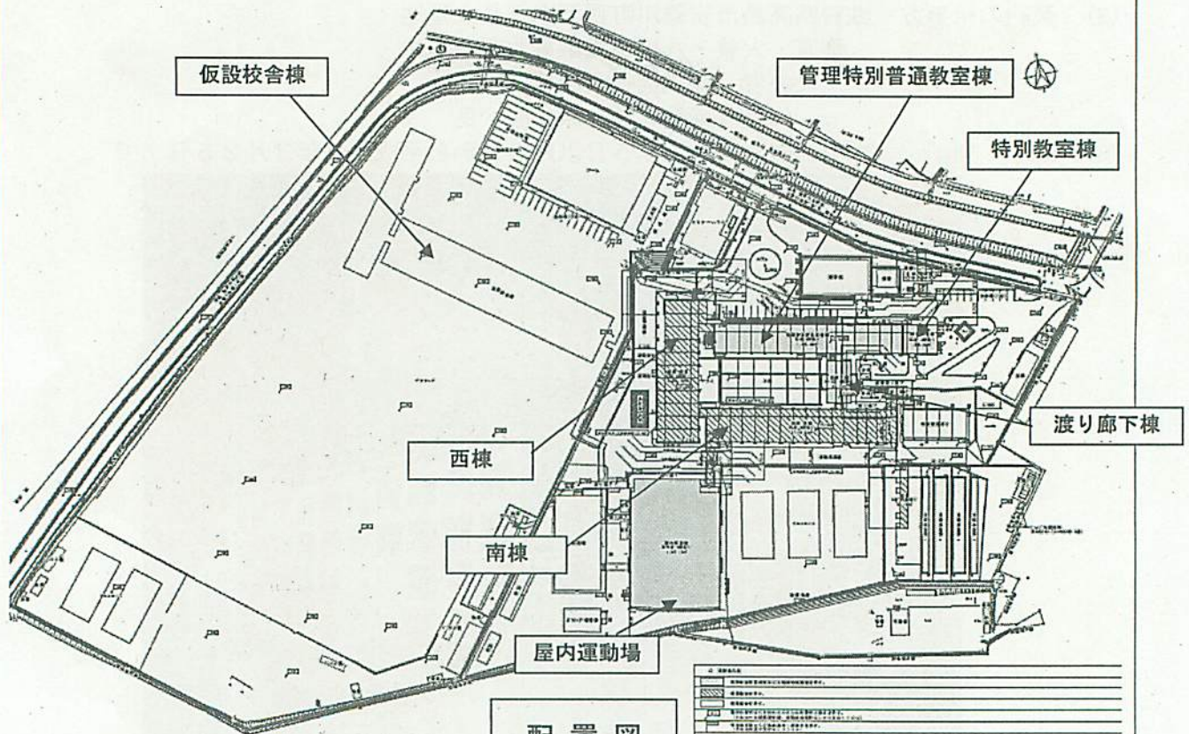
配置図
