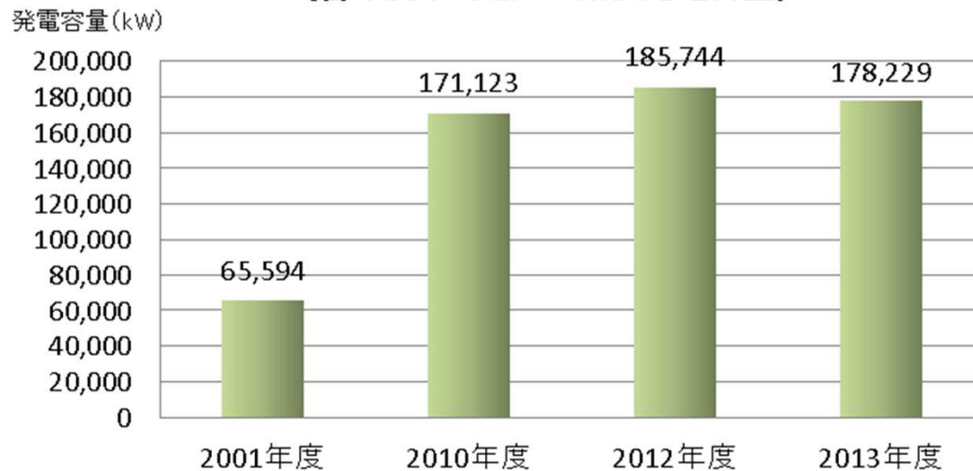
県内の天然ガスコージェネレーション導入実績 (各年度末時点での累積発電容量)
