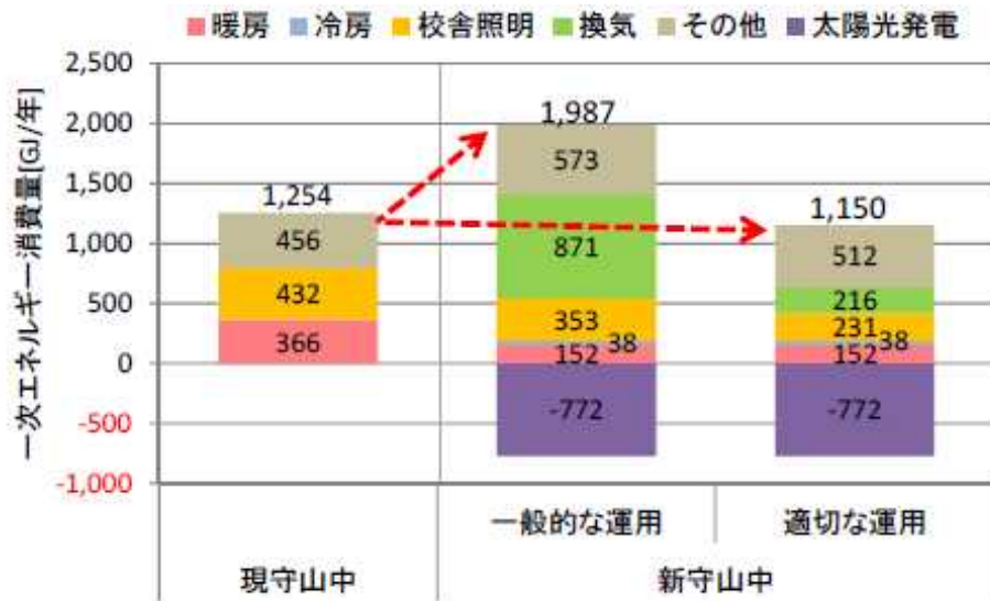
一次エネルギー消費量の試算結果
