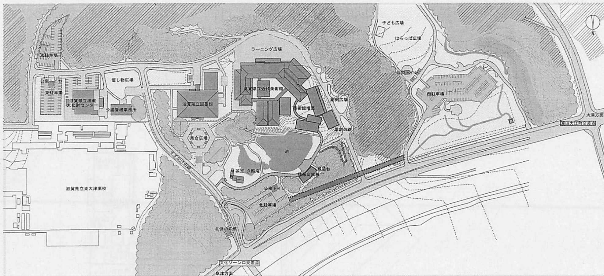
びわこ文化公園基本設計図
