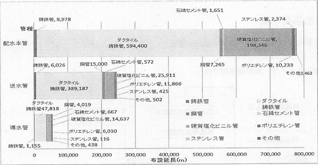
1 ■図表 3－17 上水道および水道用水供給事業の管種別布設管路の状況（m）
