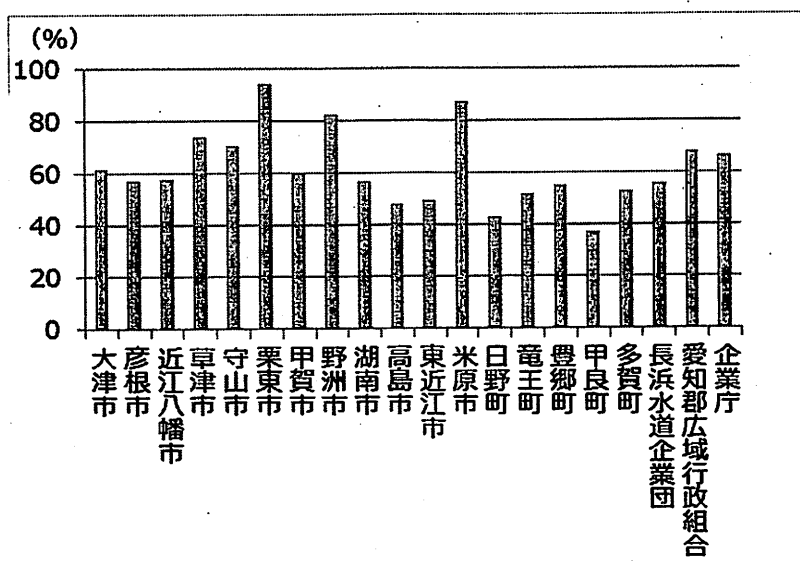
■図表 5-26 滋賀県内水道事業者の施設利用率
