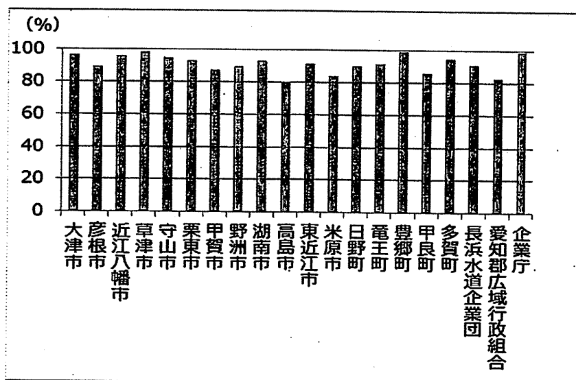
■図表5-27 滋賀県内水道事業者の有効率
