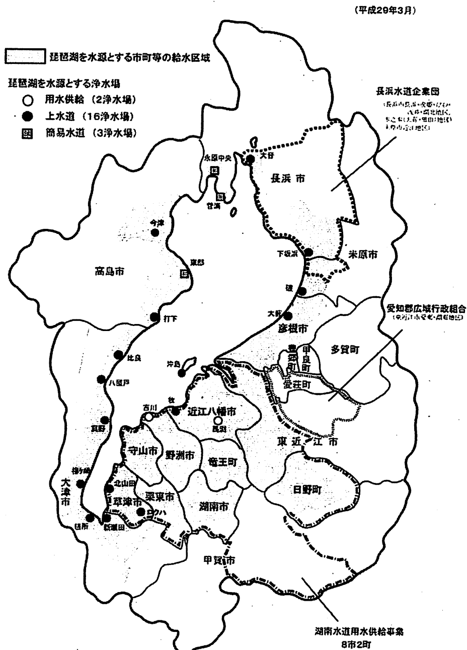
6 ■図表3-9 水道における琵琶湖水の利用状況図
