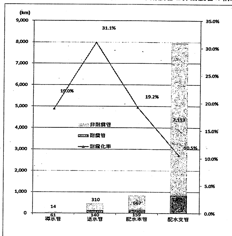
■図表5-12 滋賀県の水道管における耐震管と非耐震管の構成
