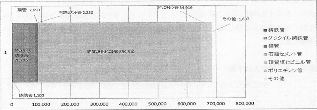
9 ■図表 3－19 簡易水道事業布設管路の状況（m）
