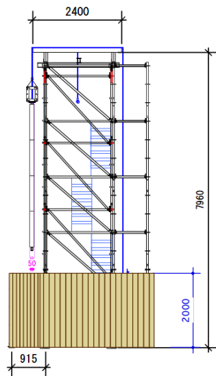
【側面図】
