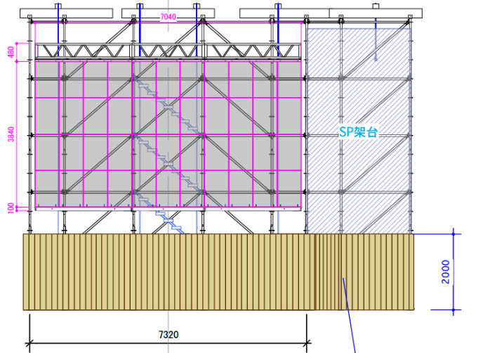
【正面図】
