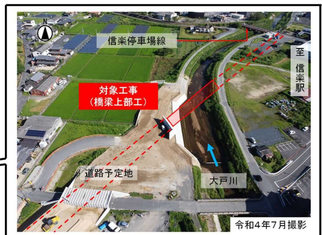
施工場所周辺拡大図
