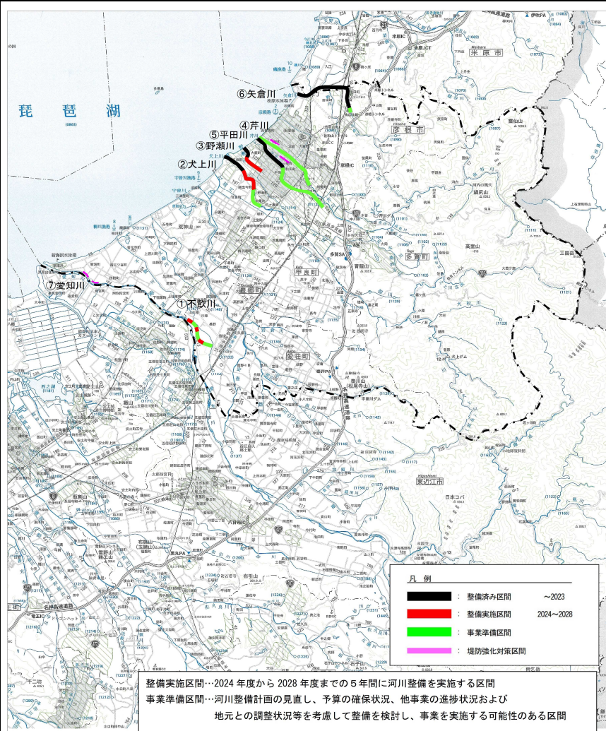
第3期計画 区間位置図(素案)
