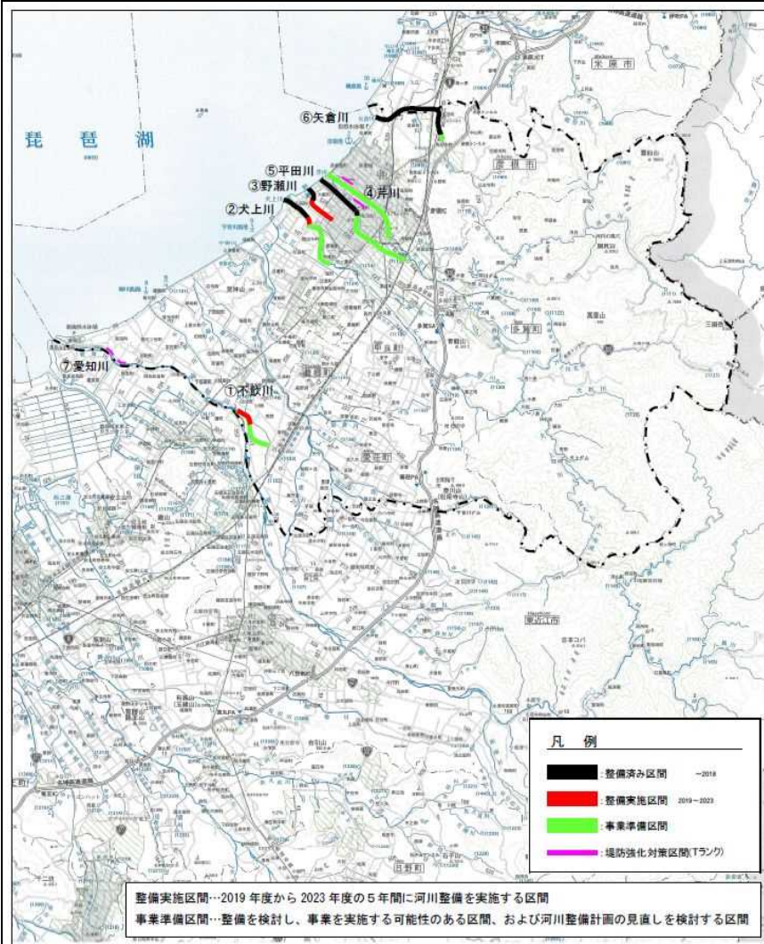
第2期計画 区間位置図
