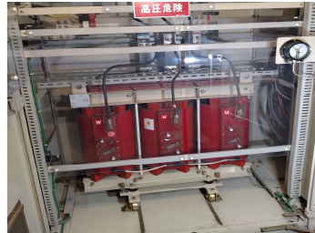
(写真5) 変圧器
