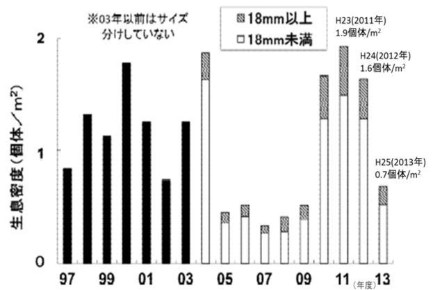
セタシジミ主要 7 漁場における生息密度の推移
