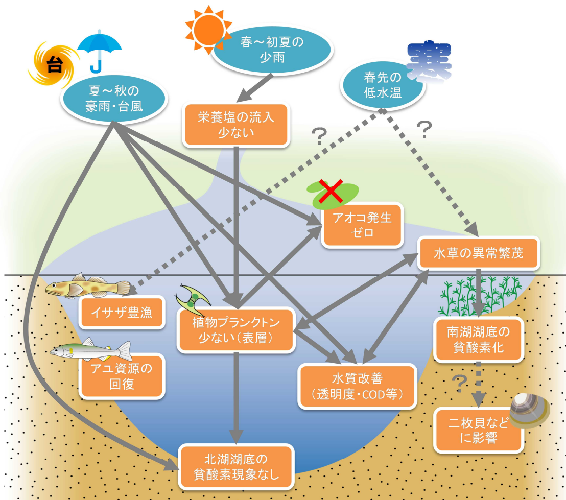
平成 26 年度に琵琶湖で生じた主要な事象の関連図
