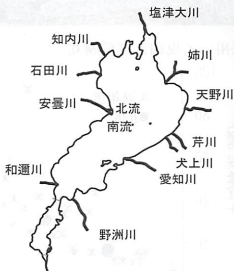
図 1 調査河川
