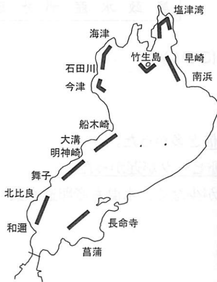
図4 調査水域(—)
