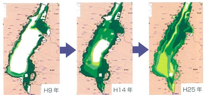
南湖における水草繁殖状況の変化 (独)水資源機構調査資料 (白色の部分は水草の植被率が0%で、色が濃い部分ほど植被率が多いことを示します。)
