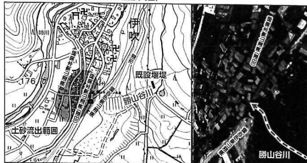
既設堰堤上流の土砂堆積状況(7月1日)
