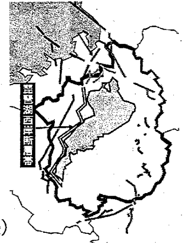
県内の主な断層帯
