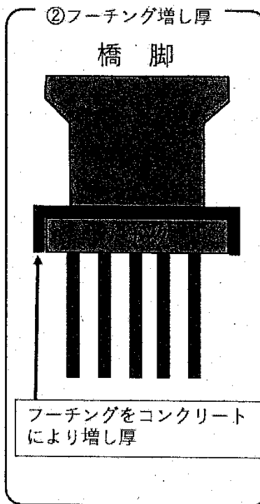
耐震工法イメージ図
