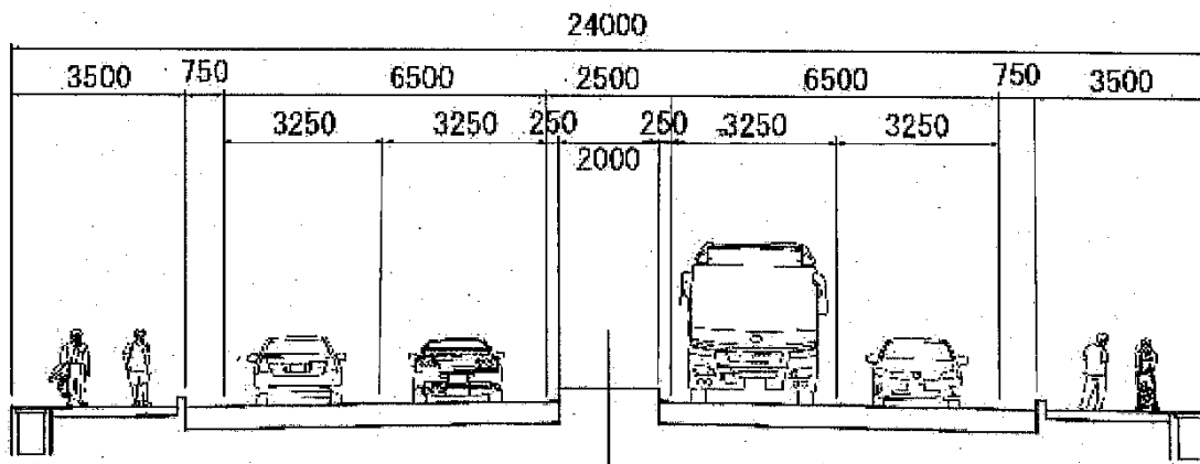
4車線拡幅(守山側)標準横断図
