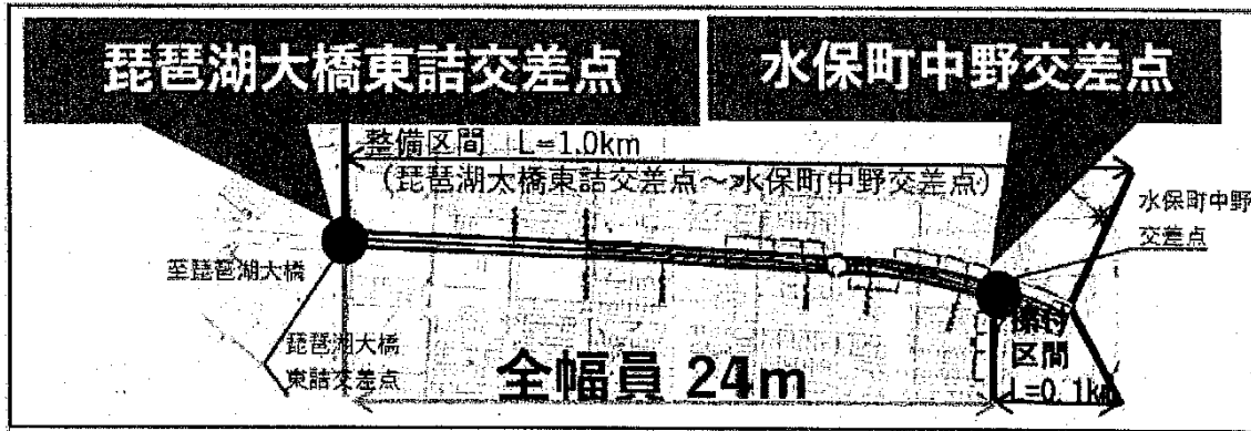
4車線拡幅(守山側)平面図
